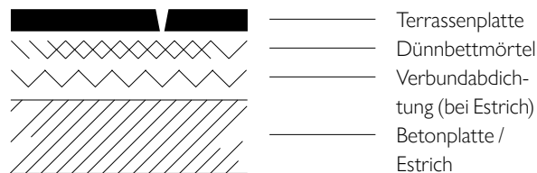
BELAGSKONSTRUKTION
